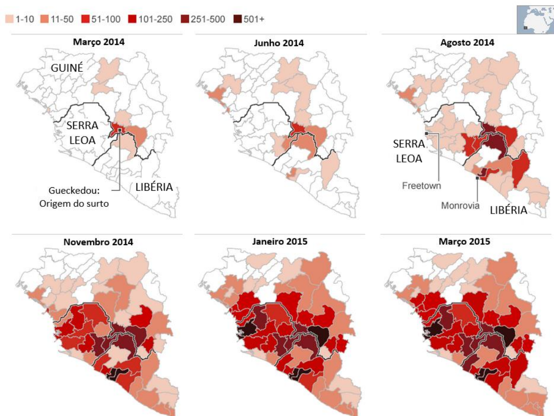
Figura 2. Evolução do número total de casos na Guiné, Serra Leoa e Libéria entre os meses de março de 2014 e março de 2015. O pico da transmissão ocorreu entre agosto e outubro de 2014. (Traduzido e adaptado de: BBC: Ebola – Mapping the outbreak, 2015) [15]
