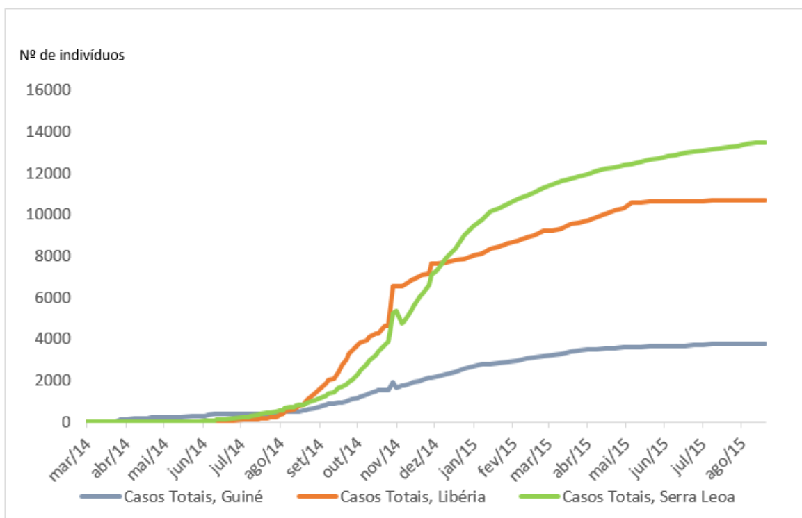
Figura 3. Número total de casos de doença provocada pelo vírus Ébola (suspeitos, prováveis e confirmados) na Guiné, Libéria e Serra Leoa, de dia 25 março de 2014 até dia 16 de agosto de 2015. n=27952. O gráfico permite avaliar a evolução da transmissão do vírus nos três países africanos mais afetados pela epidemia e concluir que a progressão da doença abrandou sobretudo a partir do mês de maio de 2015. (Retirado de: CDC - 2014 Ebola Outbreak in West Africa - Reported Cases Graphs, 2015) [18]
