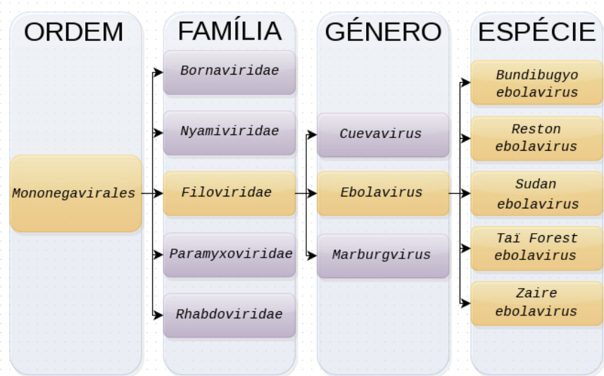
Figura 1. Classificação taxonómica do vírus Ébola, de acordo com o Comité Internacional de Taxonomia de Vírus (ICTV).
