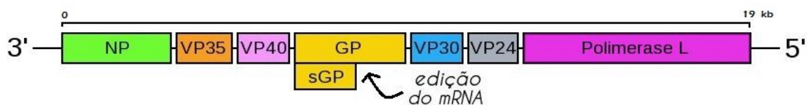
Figura 4. Genoma da espécie Zaire ebolavirus , que codifica 7 proteínas estruturais e uma não estrutural (sGP). (Traduzido e adaptado de Kanapathipillai, 2015) [8]
