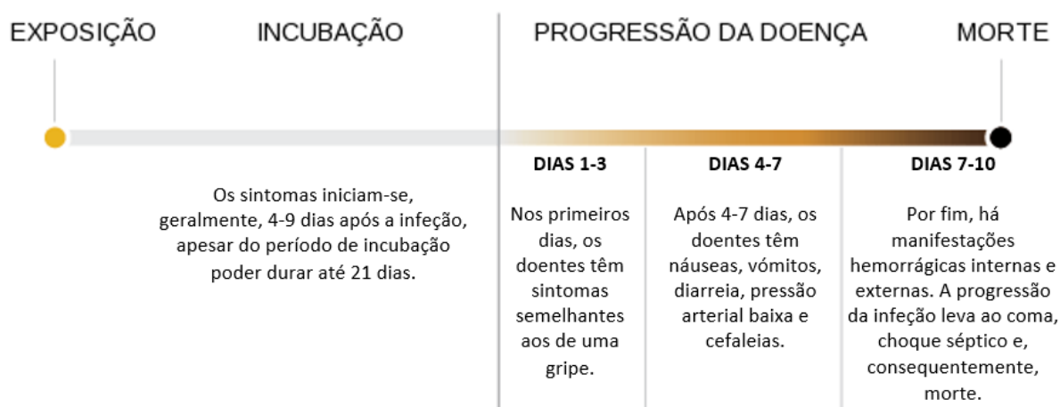
Figura 7. Etapas do desenvolvimento da doença provocada pelo vírus Ébola. (Traduzido e adaptado de: The Huffington Post - What Actually Happens When A Person Is Infected With The Ebola Virus., 2014) [32]
